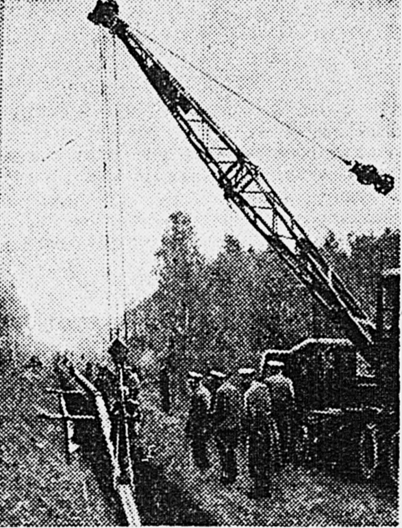
Строительство газопровода Саратов—Москва. Механизированная укладка труб.
