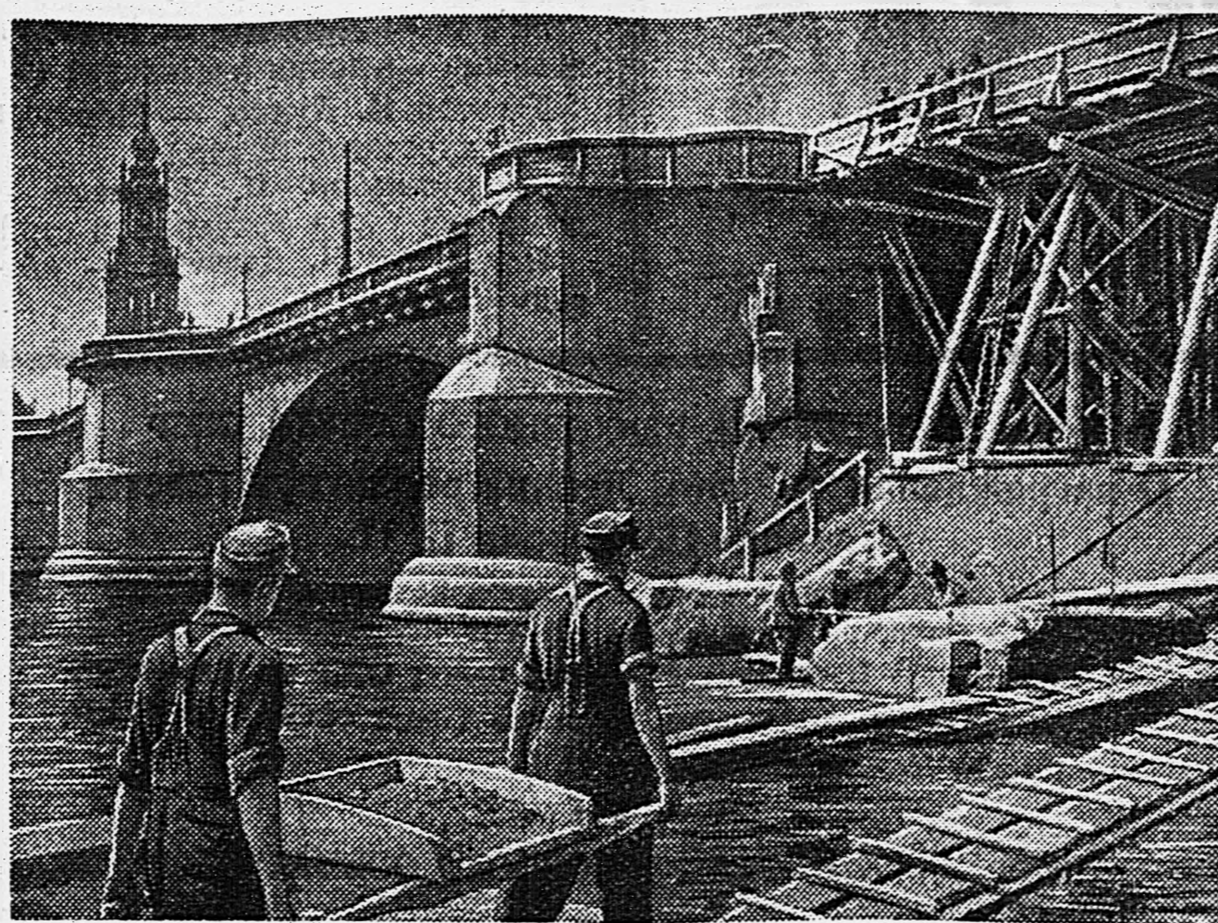
ГЕРМАНИЯ. Восстановление моста через Эльбу в Дрездене. Снимок нашего спец. фотокорр. капитана Г. Хомзара.
