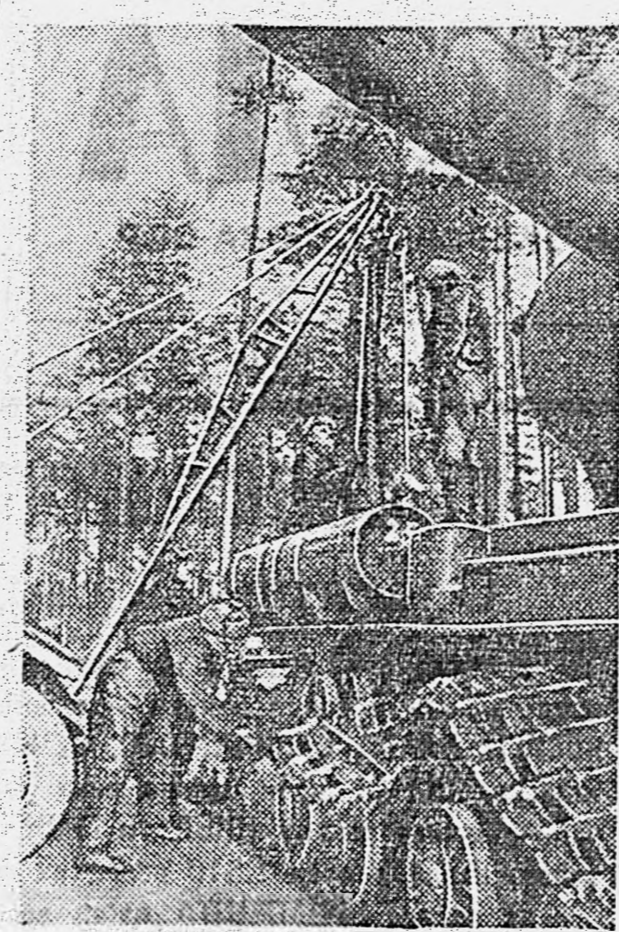
ДЕЙСТВУЮЩАЯ АРМИЯ. Ремонт танка в полевых условиях. Снимок нашего спец. фотокорр. капитана А. Капустянского.
